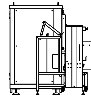
Vista da sinistra Scala: 1:20
