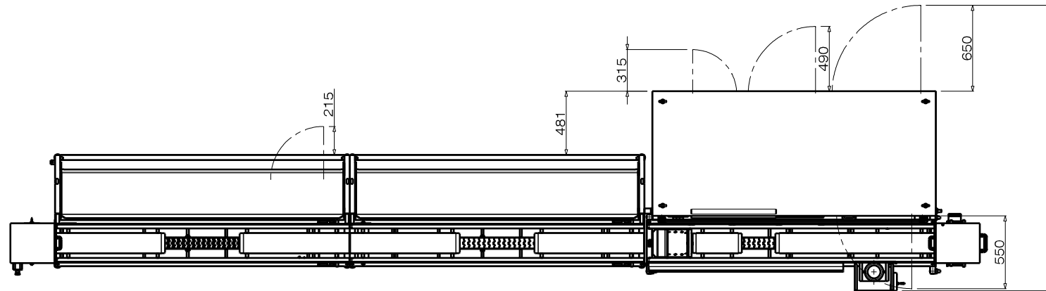
Vista dall'alto Scala: 1:20
